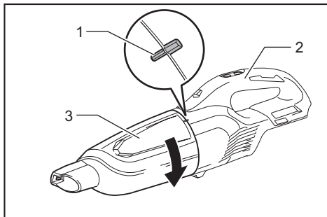
► 1. Marque 2. Poignée 3. Bac à poussière
