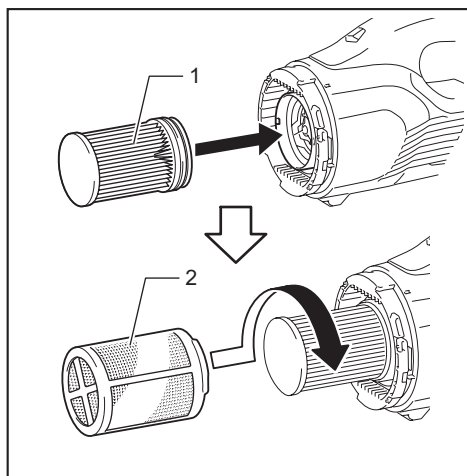
► 1. Filtre HEPA 2. Préfiltre
