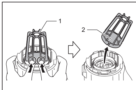
► 1. Étau 2. Filtre-éponge
